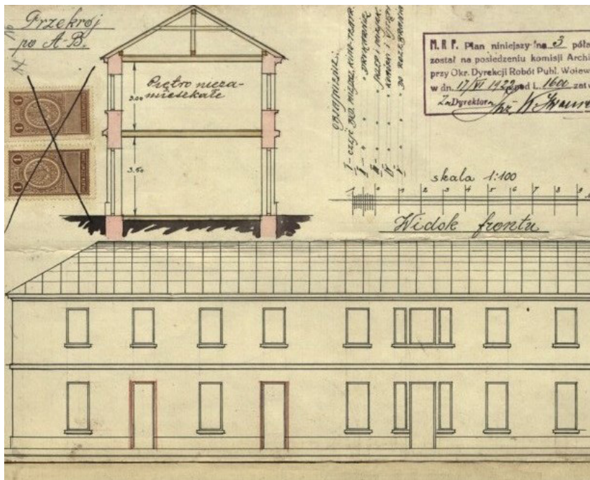
PLAN KINOTEATRU LEJZORA KAMINERA Z 1922 ROKU.
